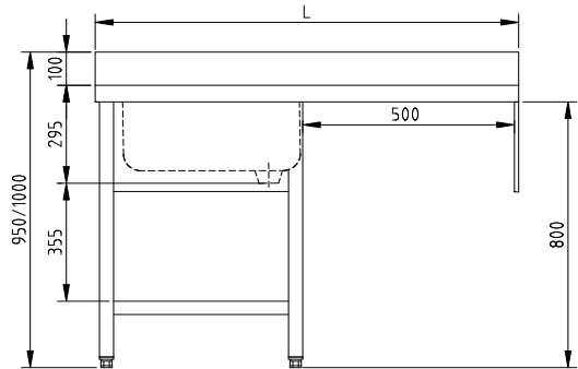
Lavavasos de hasta 500 mm de ancho
