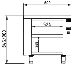
ALZADO
